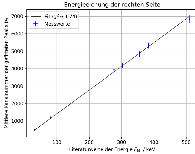
Abbildung 3: Linearer Fit der Mittelwerte b_0 der gefitteten Na- und Ba-Linien gegen die Literaturwerte der Energien E_{lit.} (Rechte Seite)
