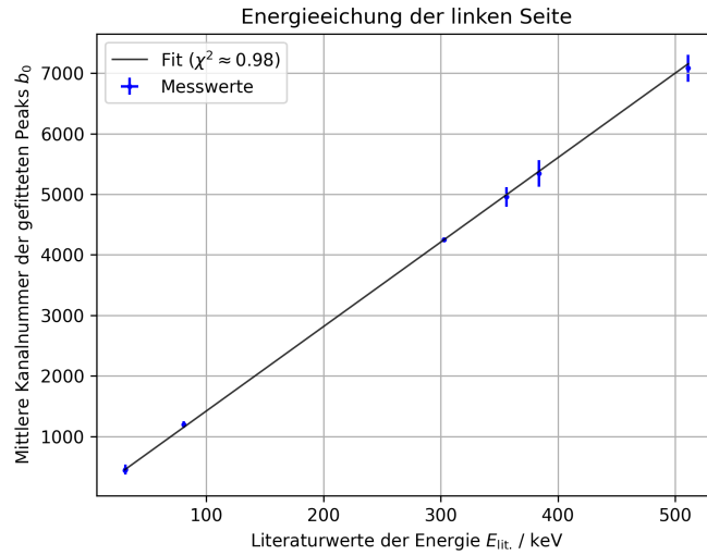
Abbildung 4: Linearer Fit der Mittelwerte b_0 der gefitteten Na- und Ba-Linien gegen die Literaturwerte der Energien E_{lit.} (Linke Seite)
