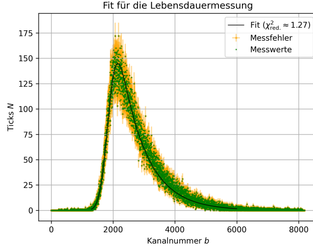
Abbildung 8: Fit der Faltungs-Funktion 10 an die Lebensdauerkurve des betrachteten ^{133}\text{Cs} -Zustandes
